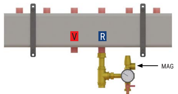
Beispiel für ungerade Anzahl an Anschlussgruppen
