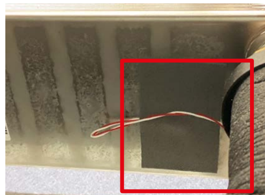
Rückansicht des Wärmetauschers mit Temperatursensor (rot)
